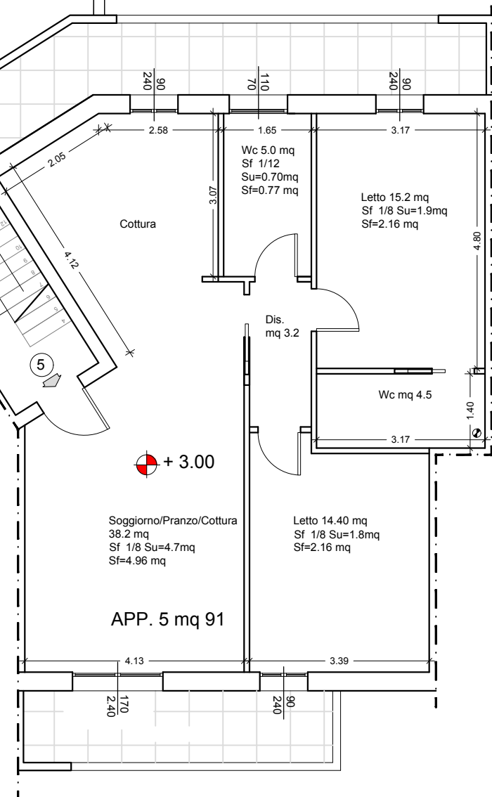
Planimetria Piano Primo
