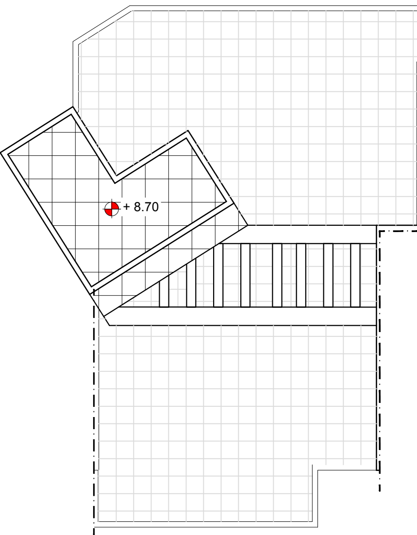
Planimetria Piano Copertura
